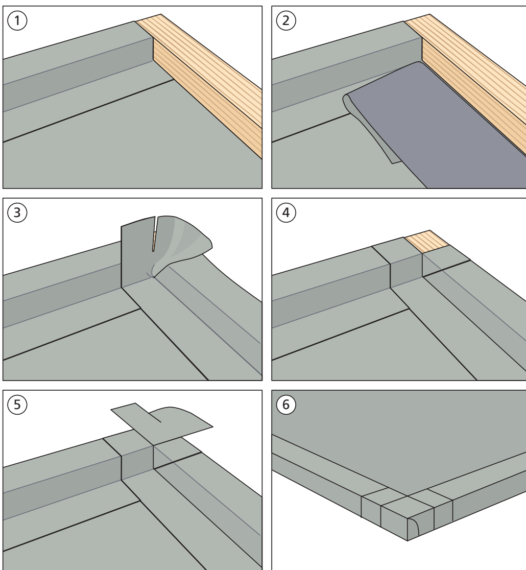
Figur 6.16: Tekking av innvendig hjørne med folie takbelegg.
