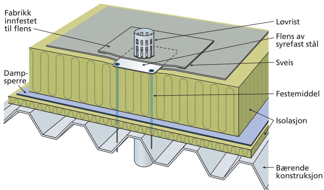
Figur 6.1 b: Prinsippskisse for tekking av sluk med folie. Folie takbelegg og sluk festes mekanisk til underlaget. Derneft sveis slukets flens til takbelegget. Mekanisk innfesting gjelder også ved bruk av innstikksluk mot asfalt takbelegg.
