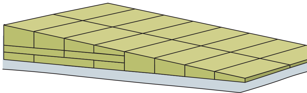
Figur 3.1: Prinsippskisse for fallopbygging med isolasjon i flere lag. Oppbyggingen kan også avsluttes med en jevntykk trykksterk toppplate.
