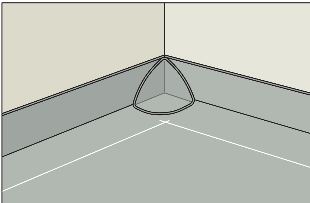
Figur 6.15: Alternativ til brettehjørne for folie takbelegg er å bruke prefabrickerte hjørner.
